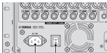
电源开关 交流电源输入
