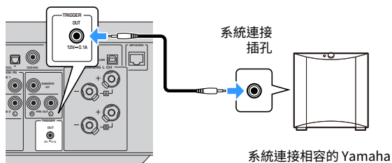
後面板
