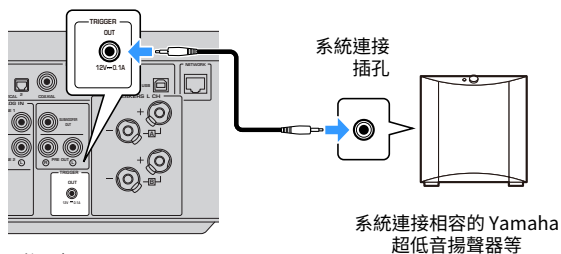
後面板
