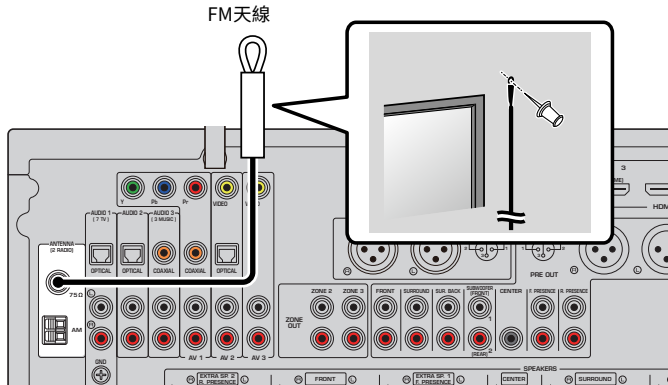
本機（後側）
