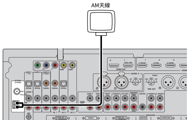
本機（後側）
